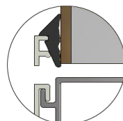
Detalj dräneringshål
